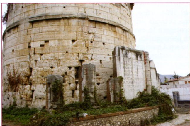
Figura 5 - Sepolcro dei Plautii, particolare con fratturazioni/fessurazioni, attacchi biologici, depositi coerenti, lato sud-ovest, foto del 2008.
