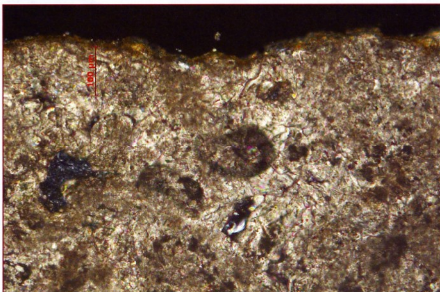
Figura 9 - Sezione sottile del campione n. 1 prelevato dal lato est del Sepolcro con evidente patina rossastra, polarizzatori incrociati
