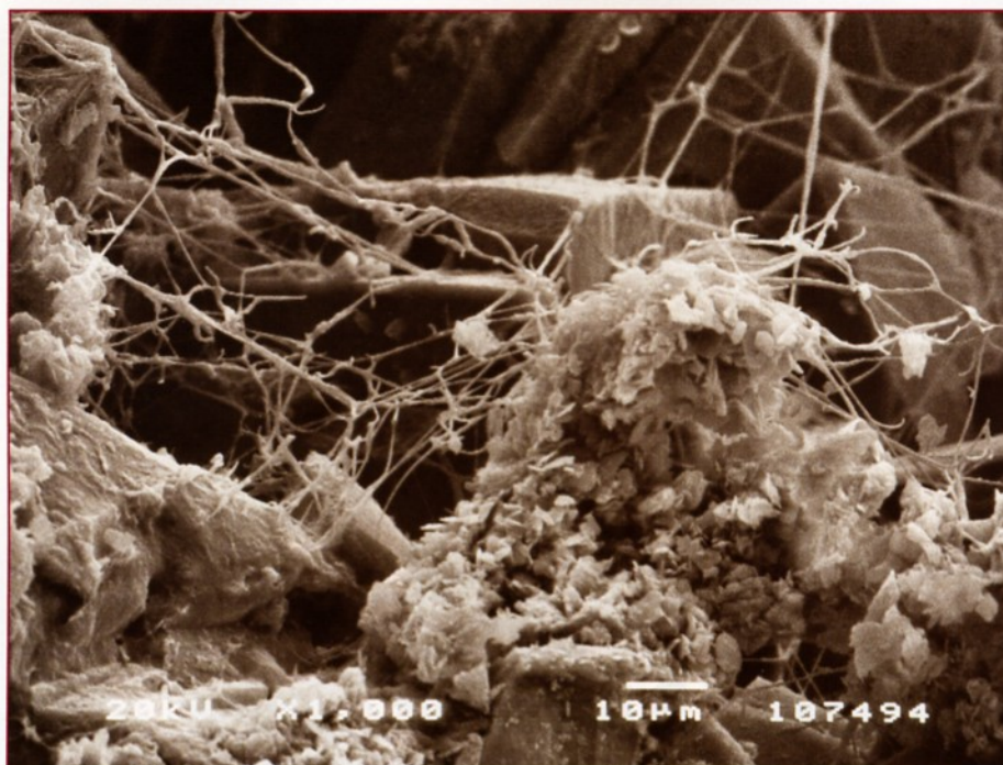
Figura 11 Immagine al SEM del campione n. 7 prelevato dal lato ovest (verso il fiume) del Sepolcro. Oltre alla presenza dei filamenti dell'alga che in certi punti sono strettamente associati al materiale lapideo, si riscontrano anche molti cristalli di gesso.
