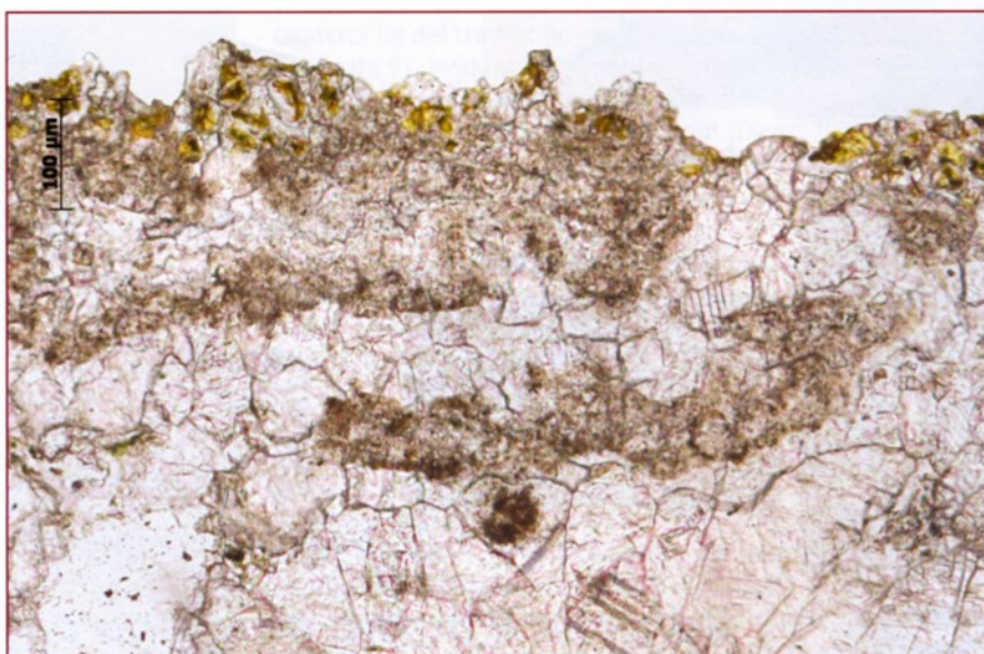
Figura 10 - Sezione sottile del campione n. 4 prelevato dal lato sud-ovest del Sepolcro con presenza di alghe verdi in superficie, polarizzatori paralleli.
