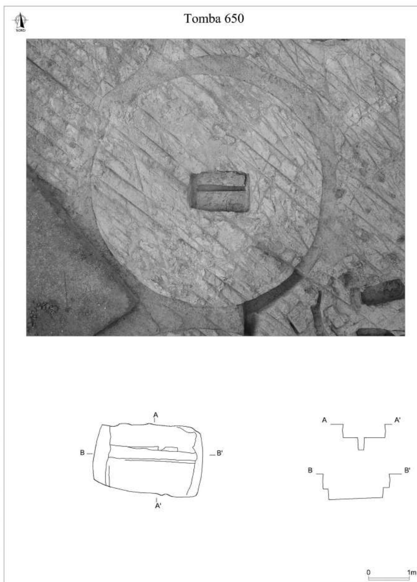
Fig. 7. Cerveteri, necropoli di Monte Abatone, tomba 650 (scavo 2021): foto da drone, pianta e sezioni (foto A. De Gemmis, ril. T. D'Anna).
