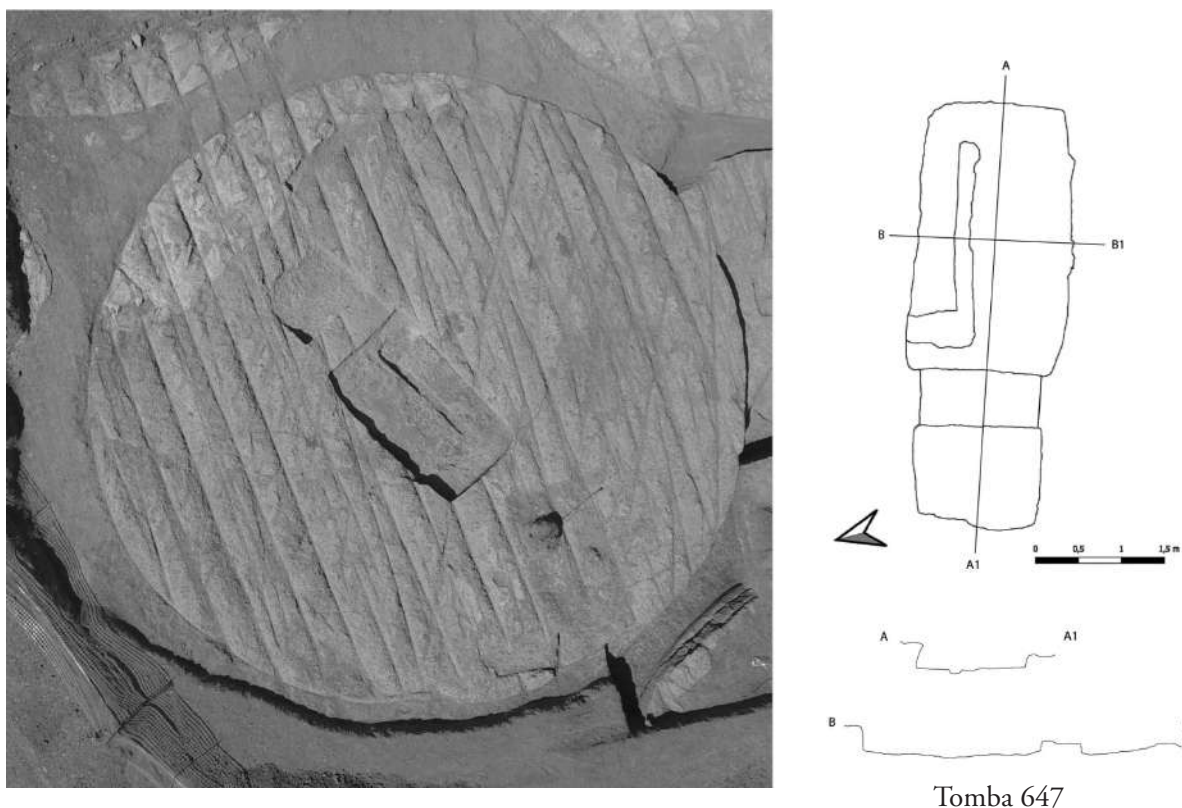
Fig. 11. Cerveteri, necropoli di Monte Abatone, tomba 647 (scavo 2021): foto da drone, planimetria e sezioni (foto e ril. L. Lucchetti).
