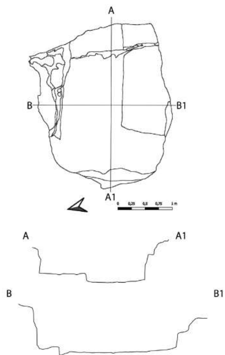
Fig. 12. Cerveteri, necropoli di Monte Abatone, tomba 651 (scavo 2021): foto, planimetria e sezioni (foto e ril. L. Lucchetti).
